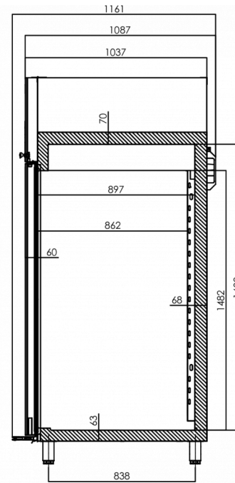
SECTION A-A
